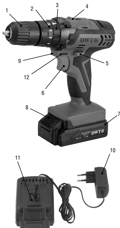
Fig. 1 – Componentes
